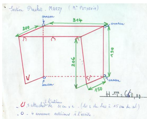
Plan de la cabane
